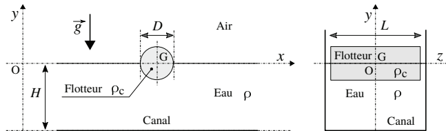
FIGURE 1 – Objet cylindrique ( \rho_c, D, L ) flottant horizontalement à la surface de l'eau ( \rho ) d'un canal (vues de face et de côté). Ces figures ne sont pas à l'échelle. En particulier, la largeur du canal n'est que très légèrement supérieure à L (l'écart est exagéré sur le schéma afin de le rendre visible).
