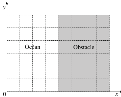
FIGURE 6 – Relief sous-marin formant une falaise verticale.
